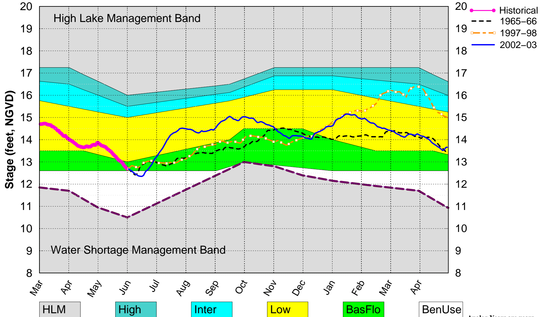
AMO Warm / El Nino Analog Years Plot PA_DPA2
