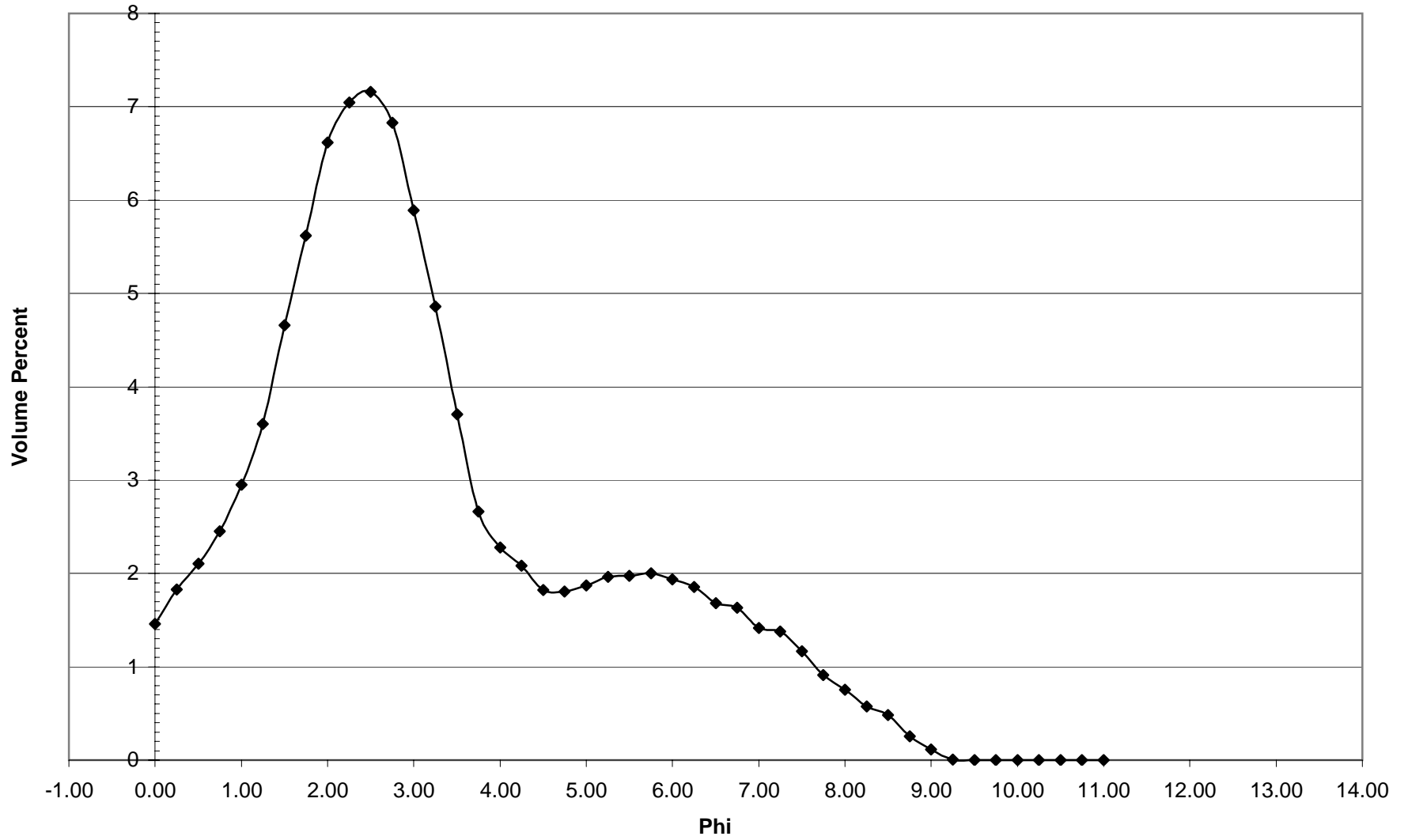
DB-58 Histogram
