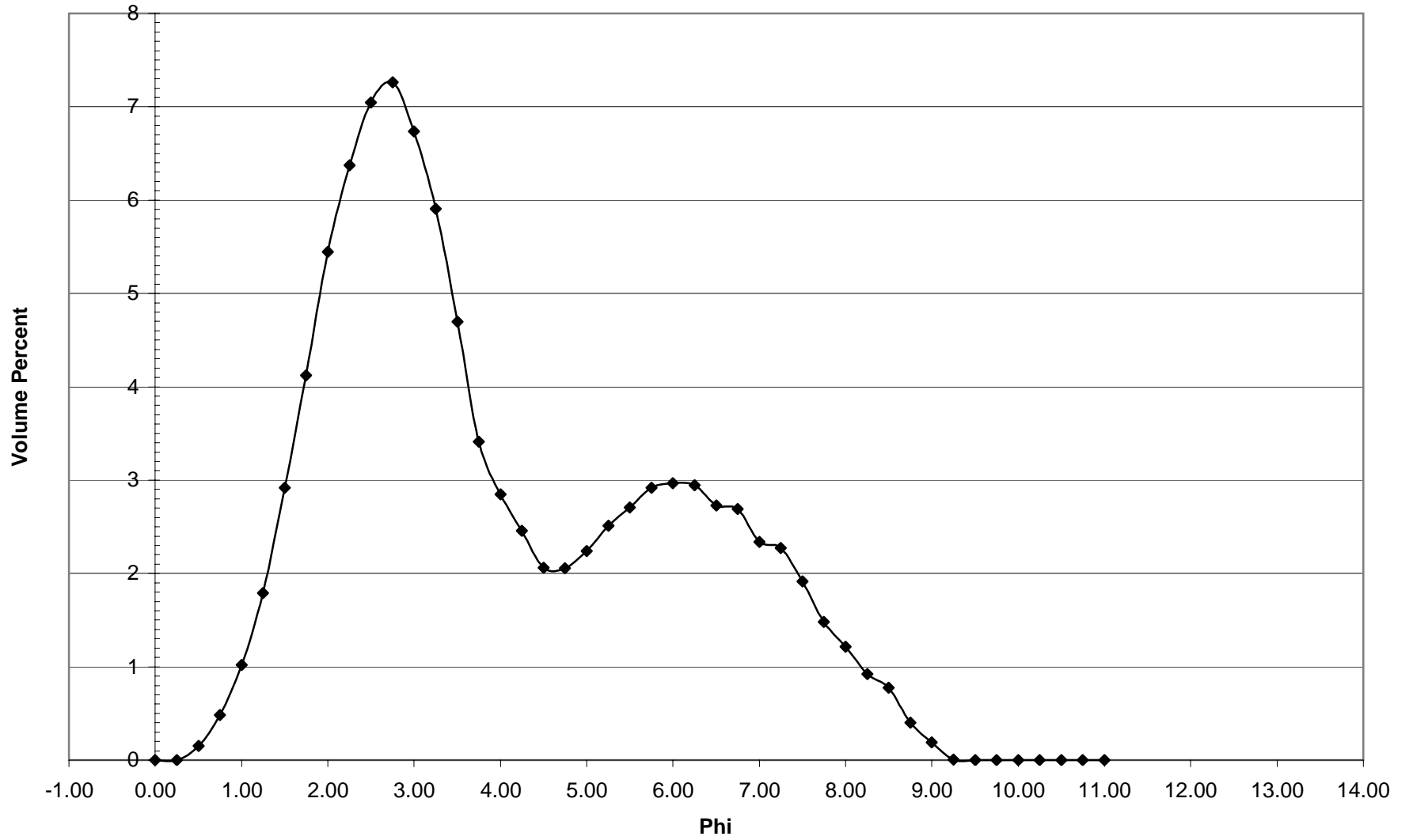
DB-60 Histogram
